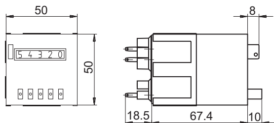
FS304 Boîtier embrochable
