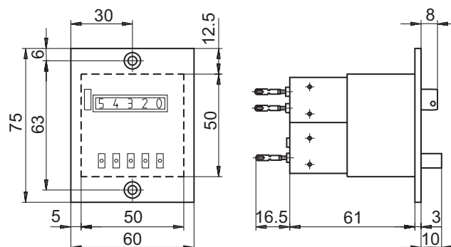
FS314 Fixation frontale par 2 vis
