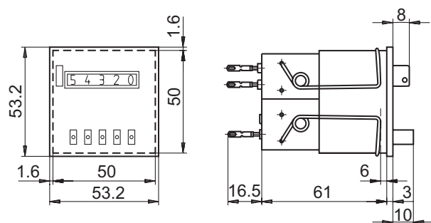
FS324 Fixation par étrier
