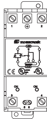
Fig. 7.A MORSETTIERA PER ISR AC
