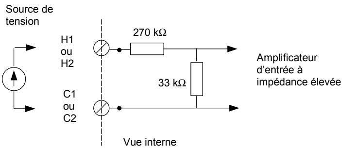
Figure 6-5 : entrée Volts
