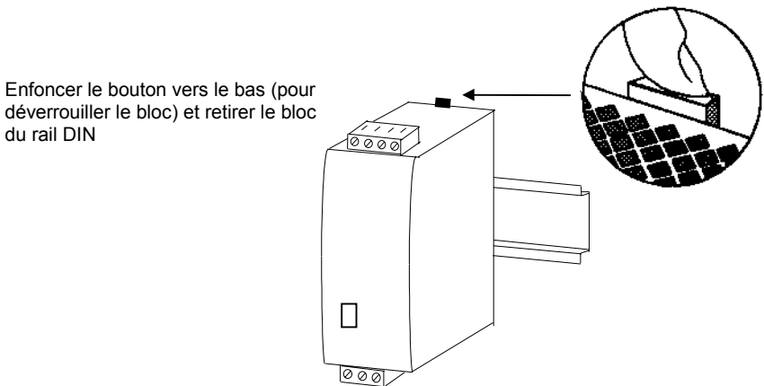
Figure 13-3 : dépose du bloc d'alimentation 2500P
