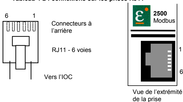
Figure 4-5 : prises et fiches RJ11 pour la configuration
