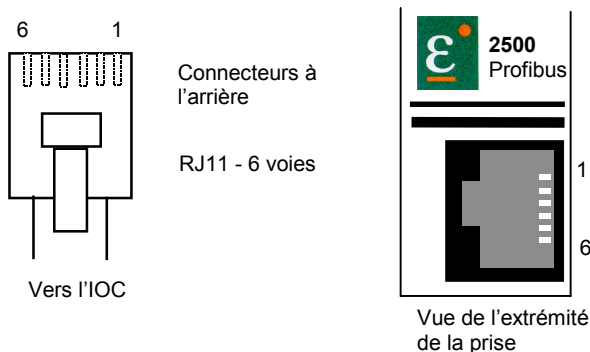
Figure 5-6 : fiche et prise RJ11
