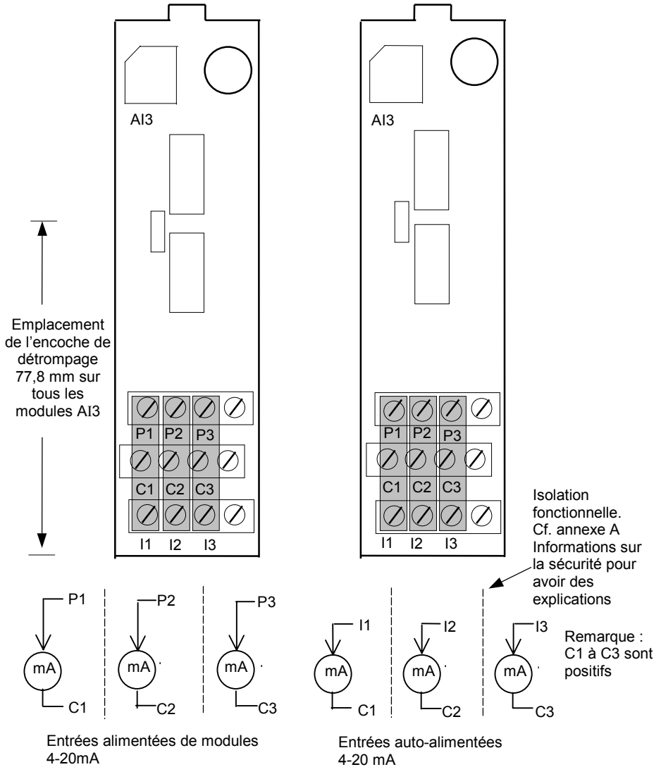
Figure 7-1 : connexions des bornes d'entrées analogiques triples
