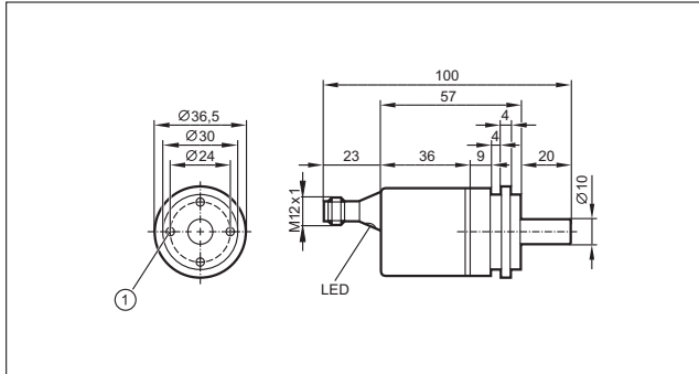
1: M4, profondeur 6 mm
