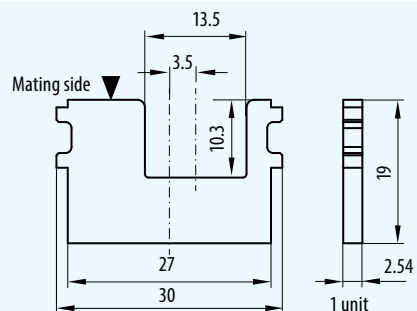
Socket
