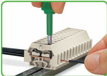
Raccordement des conducteurs – Câblage latéral, série 262
