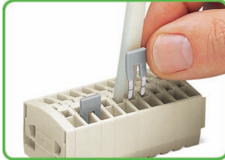
Pontage avec un peigne
