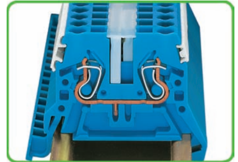
Bornes sur rail avec connexion CAGE CLAMP® COMPACT
