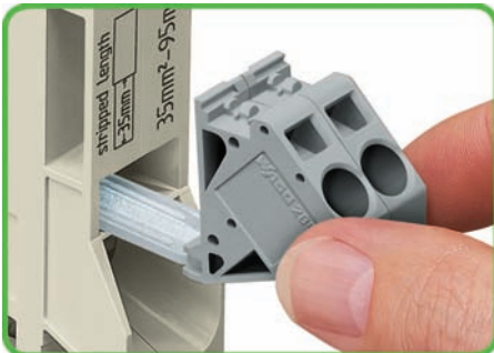
Prélèvement direct et sûr au point de l'alimentation. Enfichage de la borne de prélèvement avec le ressort relâché – sans conducteur connecté.
