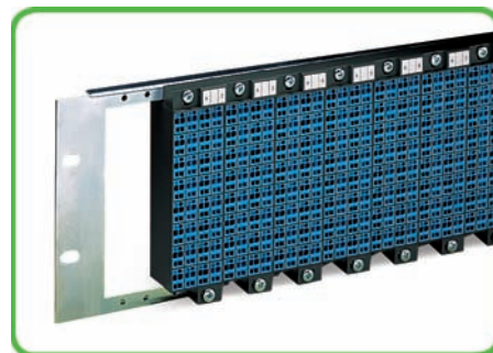
Matrices de répartition dans un rack 19"
