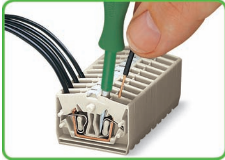
Raccordement des conducteurs – Câblage frontal, série 264
