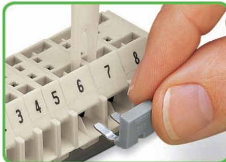
Pontage avec un peigne, série 262
