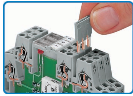
Pontage avec peigne de pontage à 3 pôles, série 859. Désormais disponible en 2 à 10 pôles.
