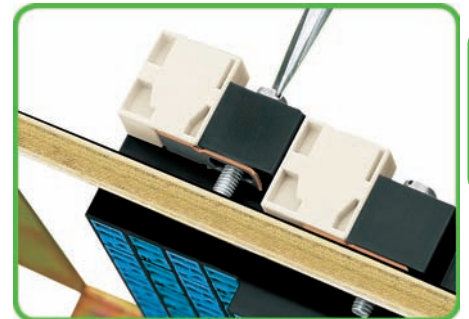
Montage d'une matrice de répartition avec une borne d'extension encliquetée. Contact direct avec le rack par la barrette
