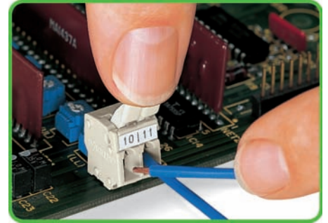
Raccordement/déconnexion des conducteurs, série 257 Actionnement manuel
