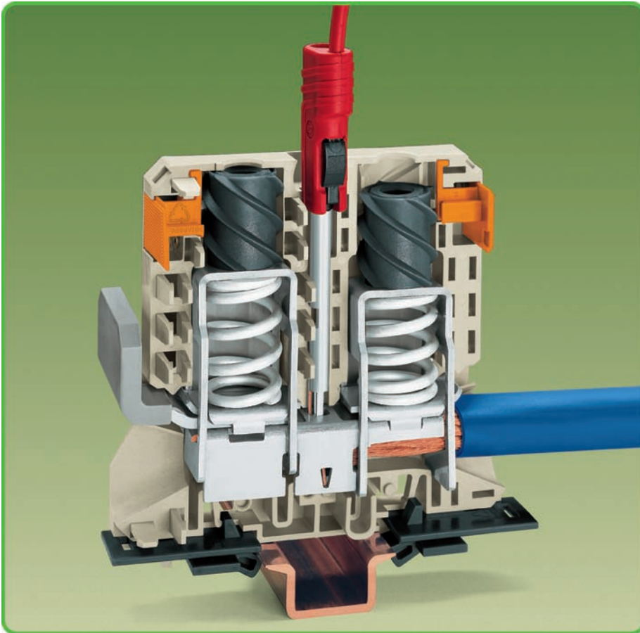
La pression de contact est distribuée de manière symétrique sur toutes les zones de contacts définies. Sécurité avec des courants de court-circuit de plus de 11,4 kA/1 sec.
