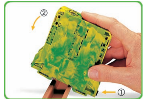
Encliquer la borne de protection sur le rail en appuyant fermement. Le pied de contact de mise à la terre crée un contact automatique avec le rail.
